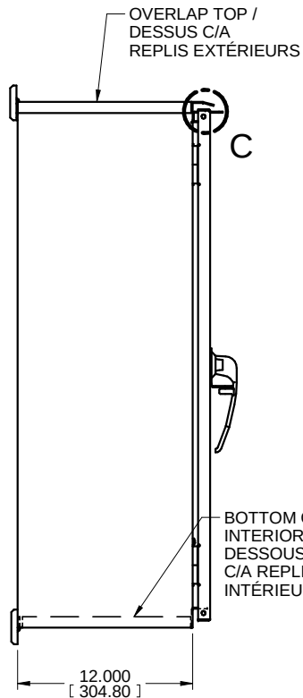
SIDE / CÔTÉ
