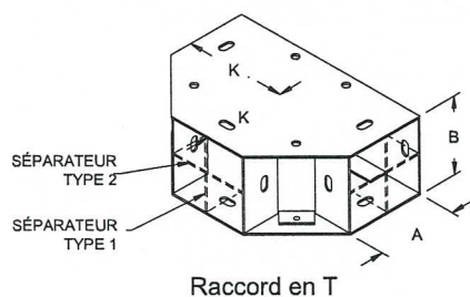
Raccord en T
