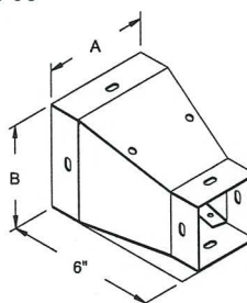
Réducteur
