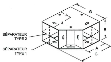
Coude 90°
