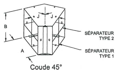
Coude 45°
