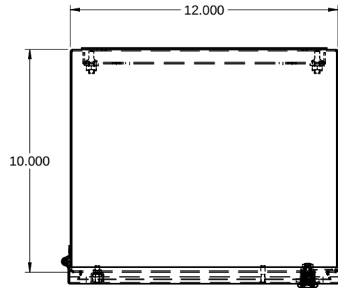
TOP / DESSUS
