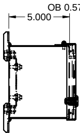
SIDE / CÔTÉ
