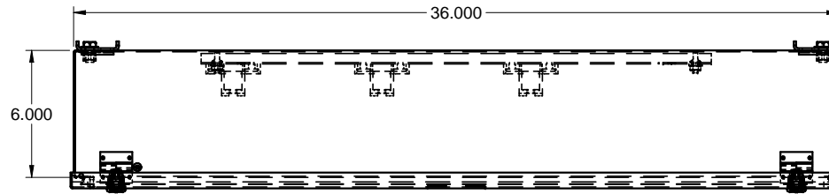
TOP / DESSUS
