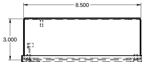
TOP / DESSUS
