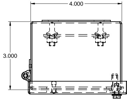
TOP / DESSUS
