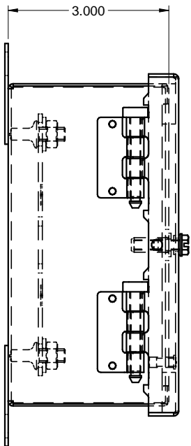
SIDE / CÔTÉ
