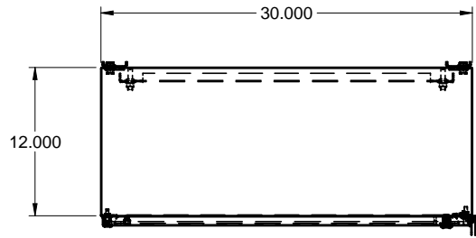
TOP / DESSUS
