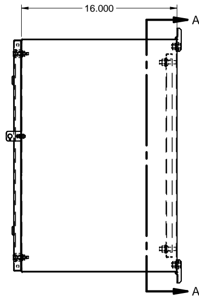
SIDE / CÔTÉ
