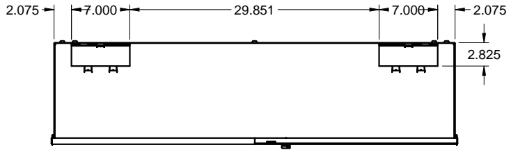
TOP / DESSUS
