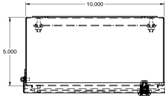
TOP / DESSUS
