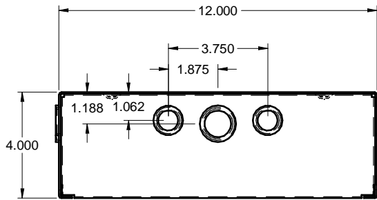
TOP / DESSUS
