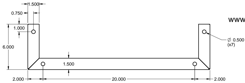
TOP / DESSUS
