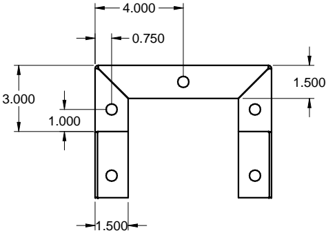
BOTTOM / DESSOUS
