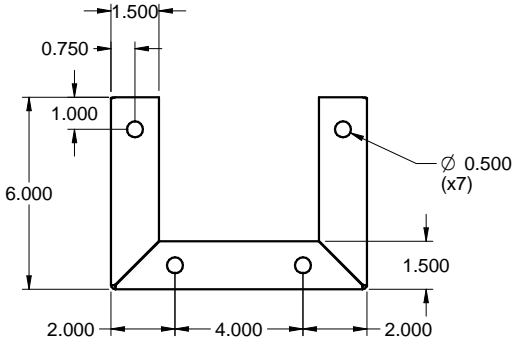
TOP / DESSUS
