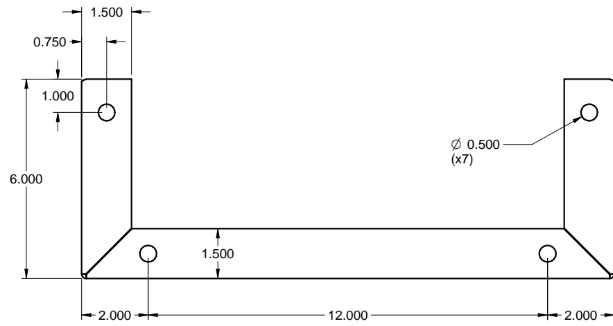
TOP / DESSUS
