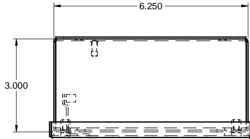
TOP / DESSUS
