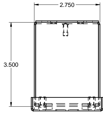
TOP / DESSUS
